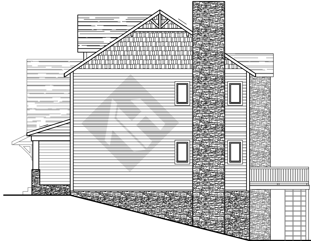
Right Elevation
