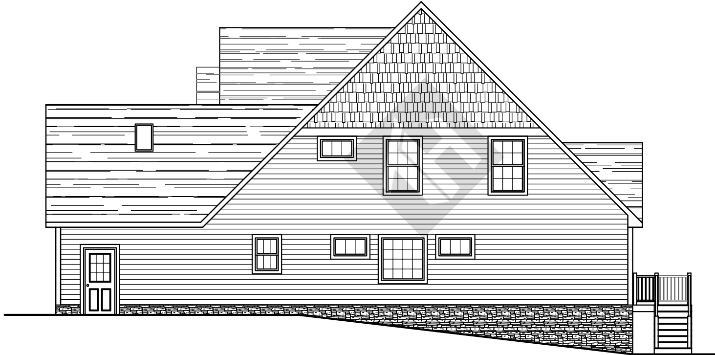
Right Elevation
