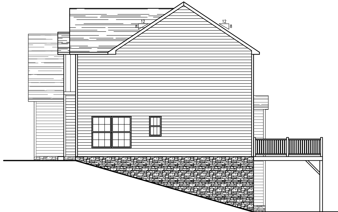
Right Elevation
