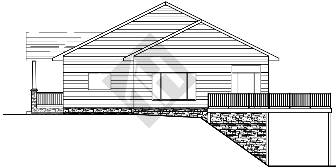
Right Elevation
