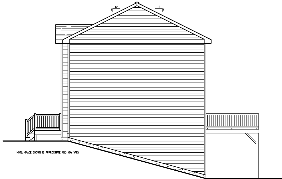
Right Elevation
