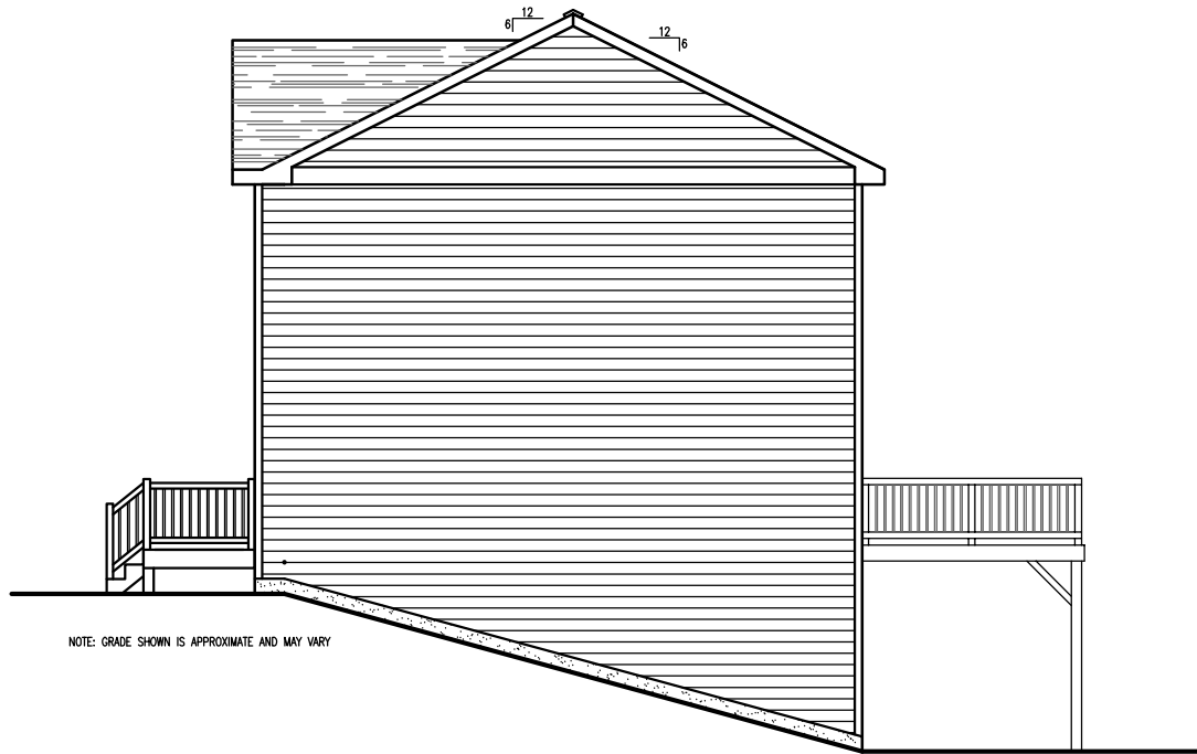
Right Elevation
