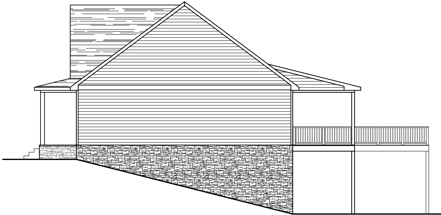
Right Elevation
